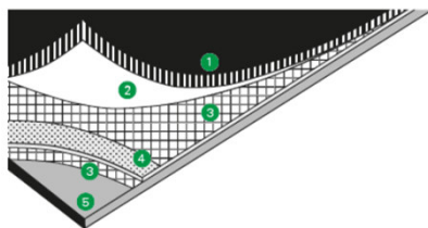
AUFBAU DER TEXTILES-RÜCKENBESCHICHTUNG
