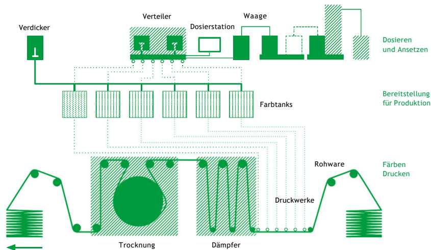
DIE FARBDOSIER- UND ANSATZSTATION
