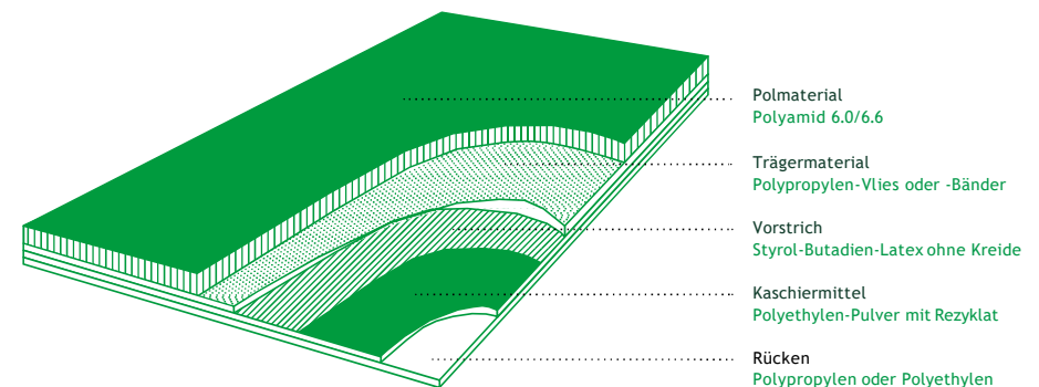
AUFBAU EINES TUFTTEPPICHS
