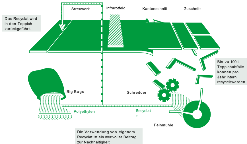
RECYCLINGKONZEPT SEIT DEN '90er JAHREN
